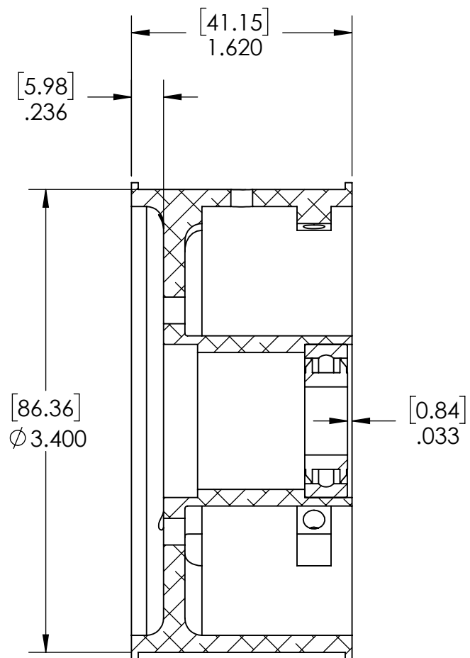
SECTION A-A
